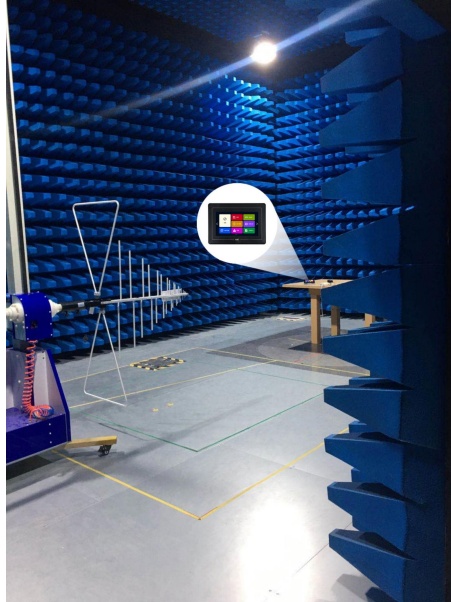
图 6-6 辐射测试图
