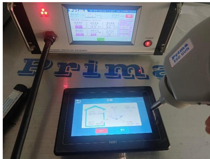
图 6-2 ESD 测试图
